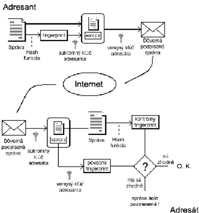
Obr. 3 Proces vytvárania elektronického podpisu
